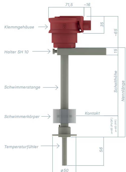
Schwimmerschalter mit einem Schaltpunkt und integriertem Temperaturfühler in LC-Ausführung / Kunststoff
