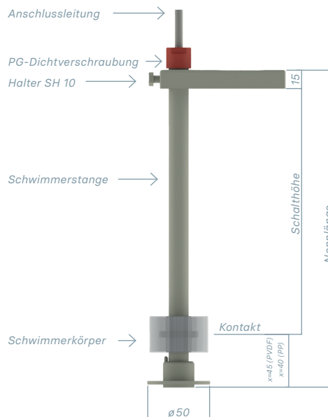
Schwimmerschalter mit einem Schaltpunkt in PG-Ausführung / Kunststoff
